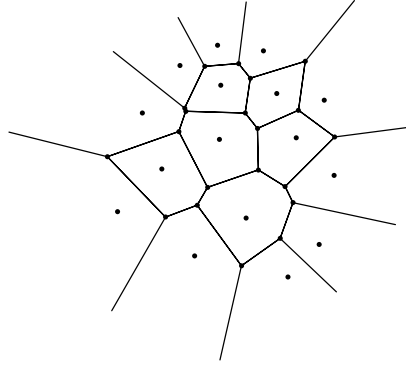
Fig. 15.30. A Voronoi diagram.
