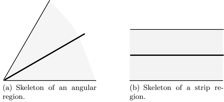
Fig. 4.3. The examples of Lemma 4.6.
