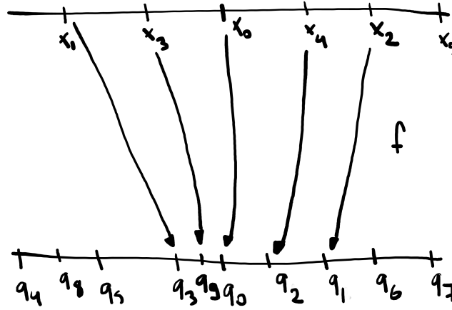
Figura 2.5: Construindo o isomorfismo
